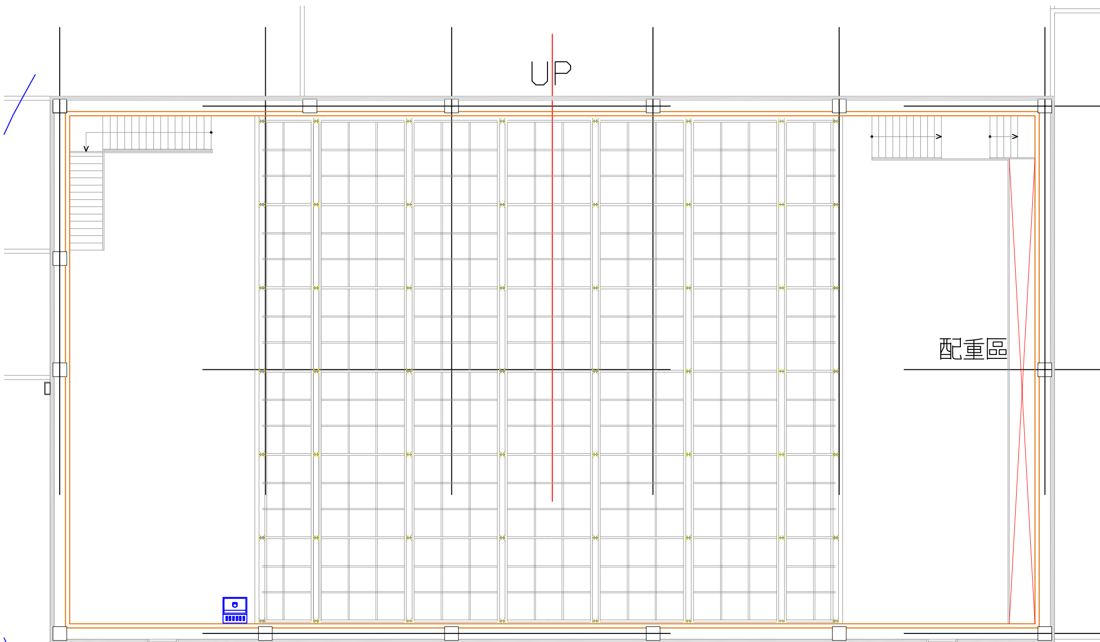
燈光系統7F 吊具鋼棚迴路圖
