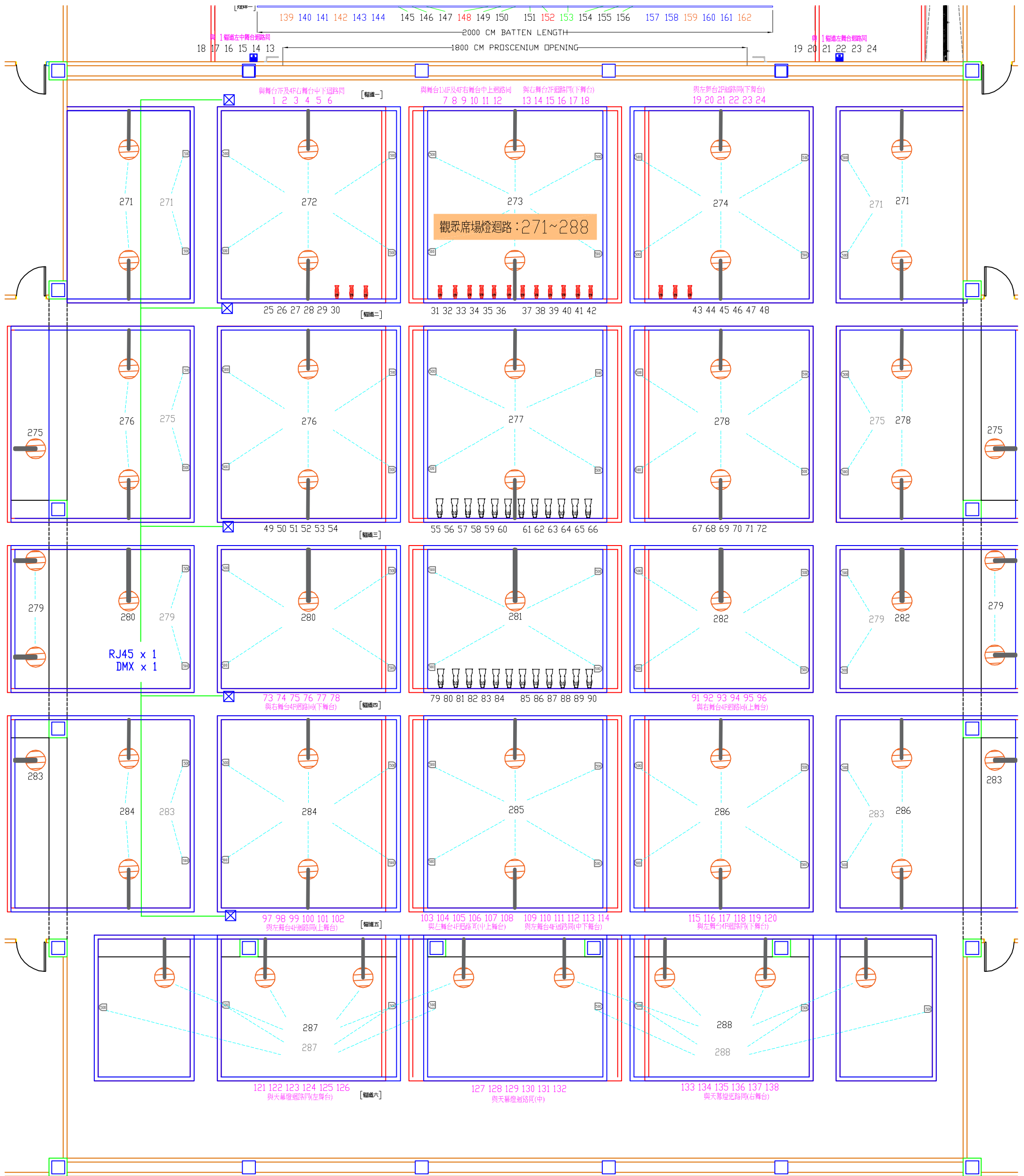
貓道燈光迴路及基本配置平面圖
