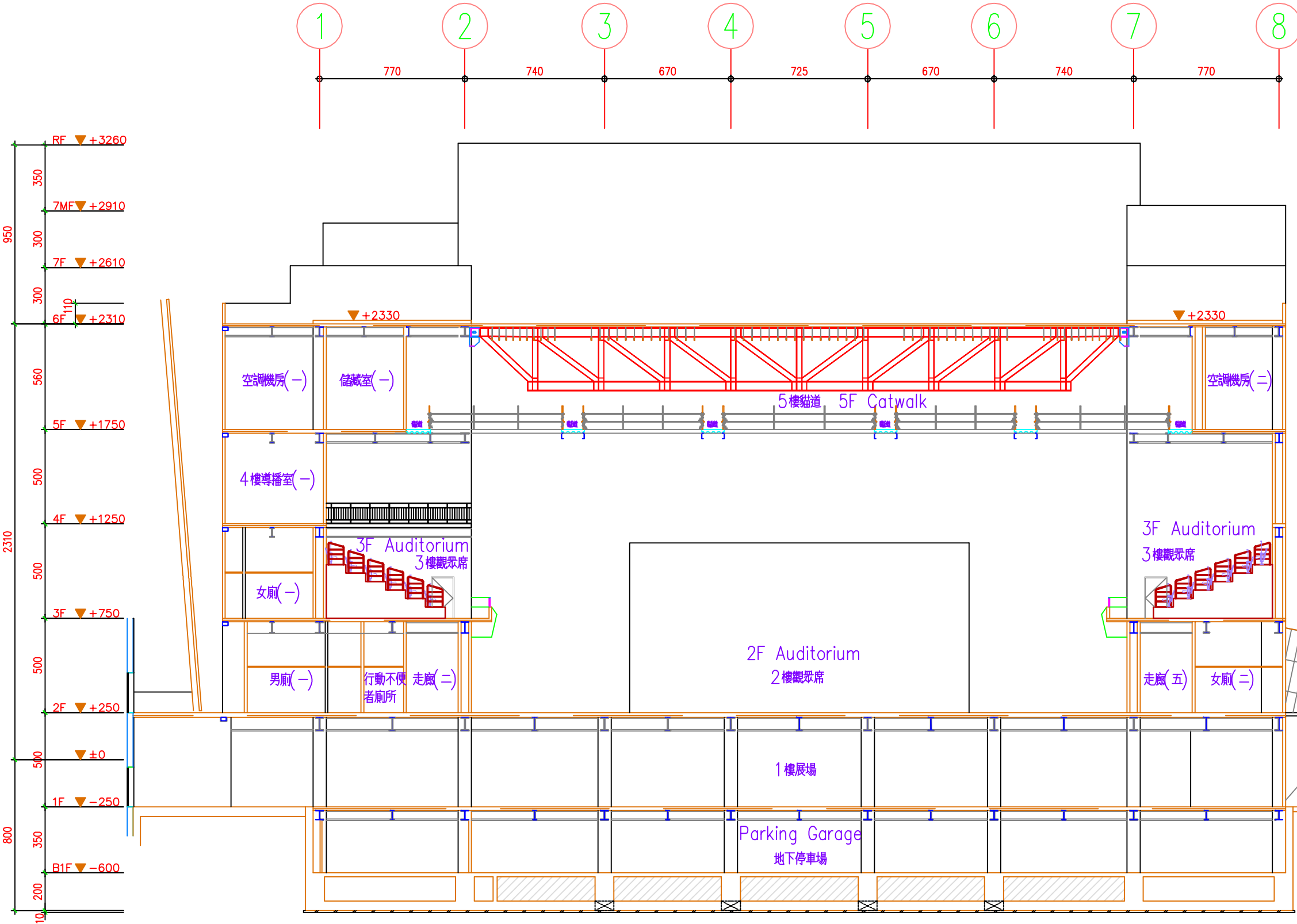
2 橫向總剖面圖(二) Cross Section(2)
