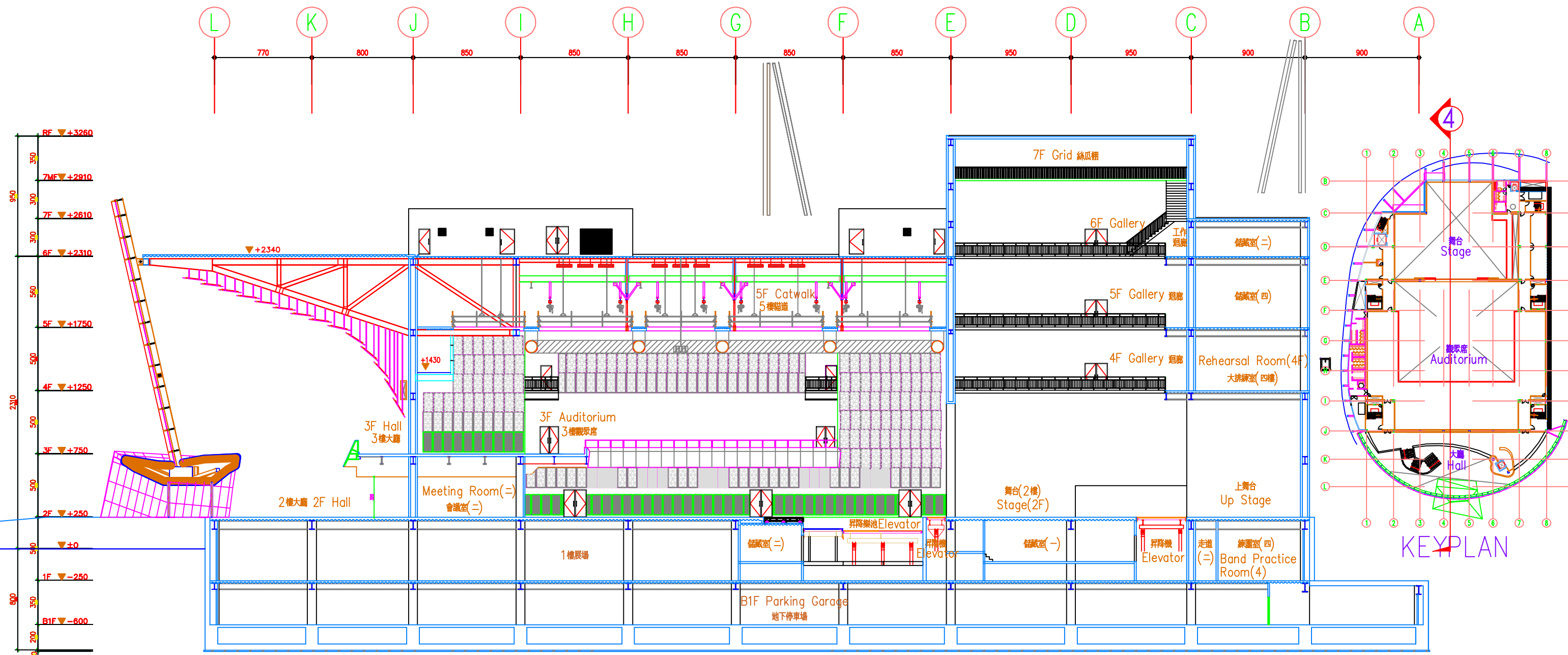
4 縱向總剖面圖 Longitudinal section
